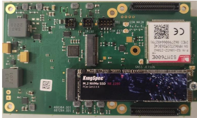
Рис.4 Установленный SSD-диск в ПАК
